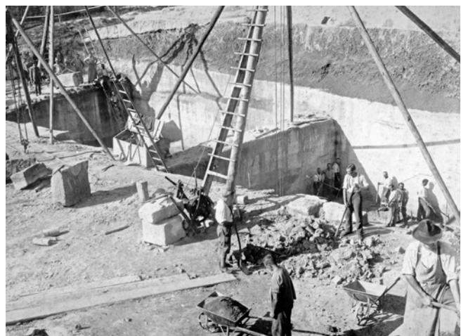
In vier Gruben in Buchenbühl wurde ohne größere Maschinen Sandstein abgebaut und mit einer Feldbahn zu den Baustellen transportiert. Das so gewonnene Baumaterial war billiger als Ziegelsteine. Fotografie 1919.
